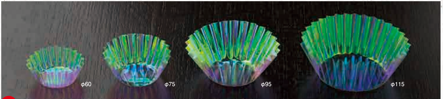
New ティスティークップ オーロラ 厚口(φ60・φ75・φ95・φ115) φ60: φ45×H15mm 底径φ30mm (500枚×10)×6箱 φ75: φ55×H22.5mm 底径φ30mm (500枚×10)×6箱 φ95: φ75×H27.5mm 底径φ40mm (500枚×10)×6箱 φ115: φ83×H30mm 底径φ55mm (500枚×10)×6箱
